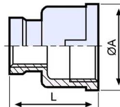
Copla de Unión - hilo NPT, F/F - A351, 316L
