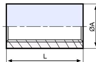
Copla de Unión - hilo NPT, F/F - A351, 316L
